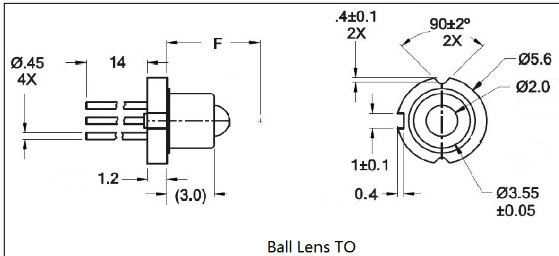
图 2.1 器件外观参数
